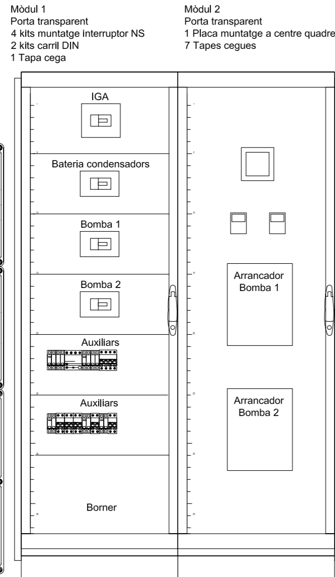
Armarí Schneider Prisma Plus P IP55 2 mòduls 650 x 2000 x 600mm Zòcal 100mm
